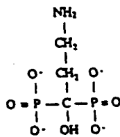
Pamidronate
